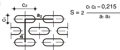
FORI OBLUNGHI ALTERNATI STAGGERED SLOT HOLES TROUS OBLONGS ALTERNÉS
