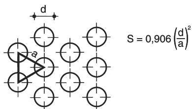
FORI TONDI A QUINCONCE A 60° 60° STAGGERED ROUND HOLES TROUS RONDS À 60°
