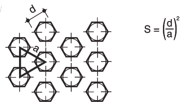
FORI ESAGONALI A QUINCONCE A 60° 60° STAGGERED EXAGONAL HOLES TROUS HEXAGON. EN QUINCONCE À 60°
