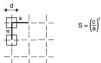
FORI QUADRI IN LINEA A 90° 90° IN LINE HOLES TROUS CARRÉS EN LIGNE À 90°
